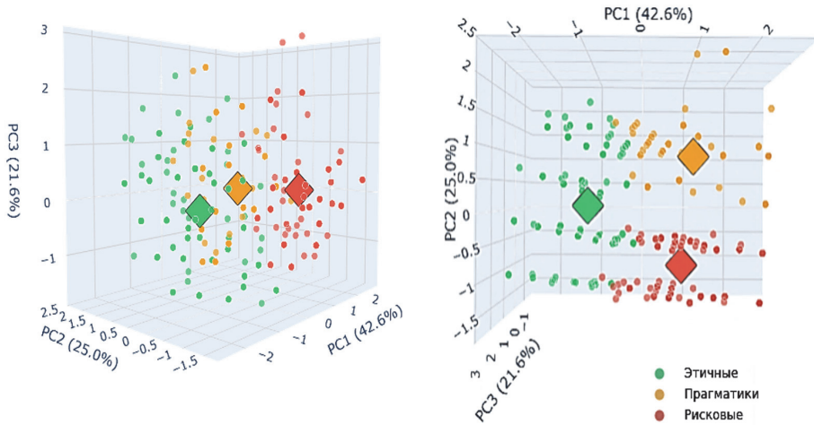
Рис. 3. 3D PCA-графика: распределение нормализованных средних значений по кластерам
